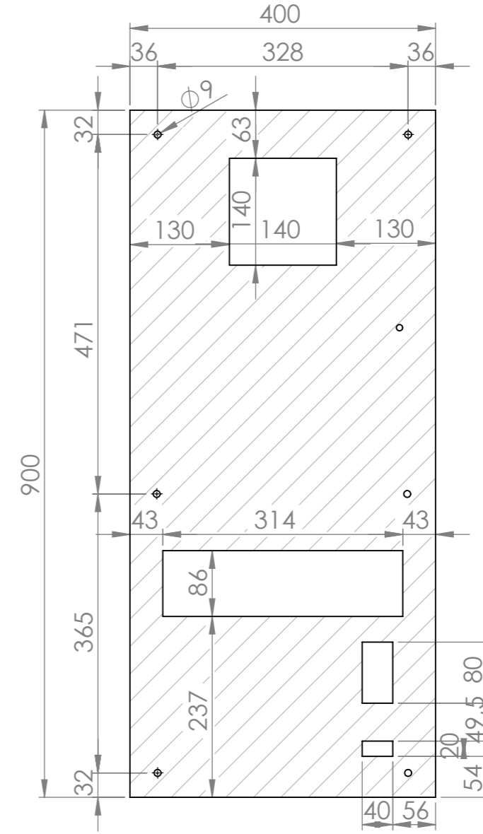
KESİM ŞABLONU
