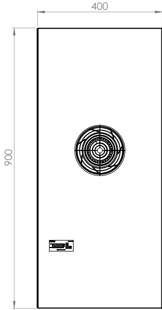
ÖN GÖRÜNÜŞ
