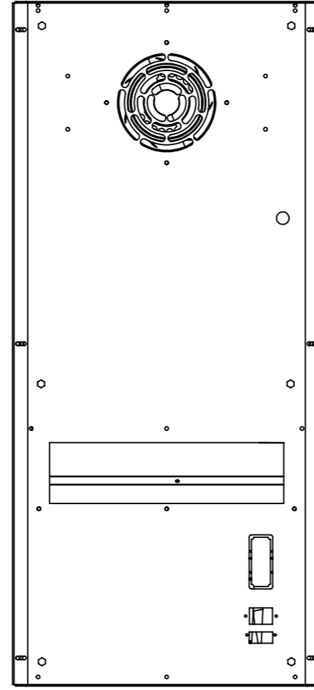
ARKA GÖRÜNÜŞ
