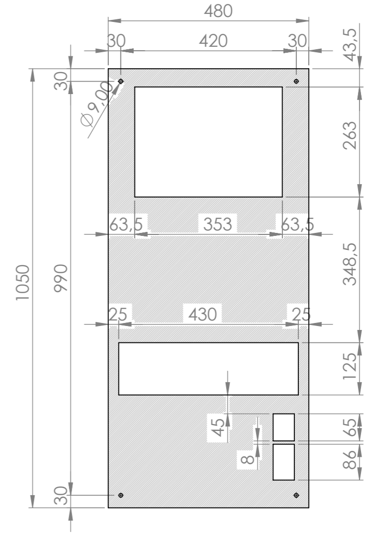
KESİM ŞABLONU
