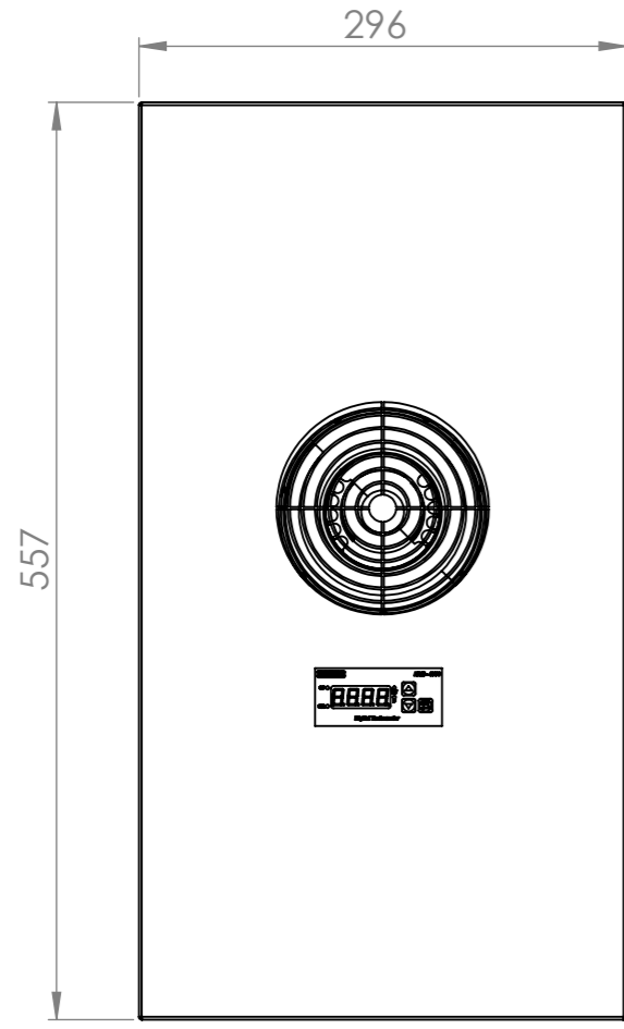
ÖN GÖRÜNÜŞ
