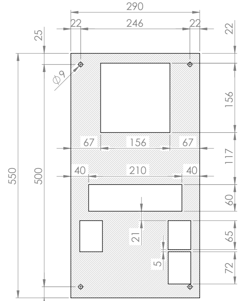
KESİM ŞABLONU
