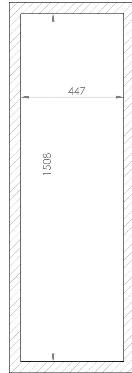
KESİM ŞABLONU
