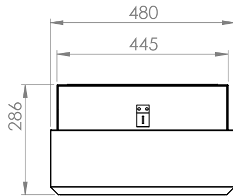
ÜST GÖRÜNÜŞ
