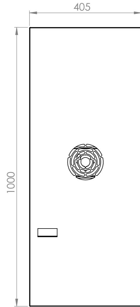
ÖN GÖRÜNÜŞ
