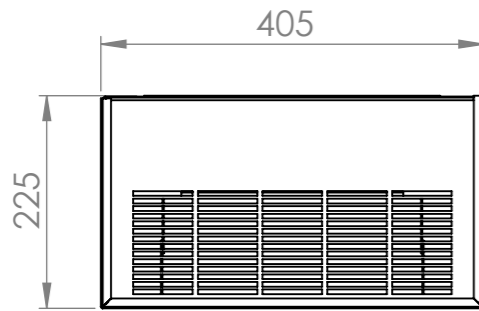
ÜST GÖRÜNÜŞ
