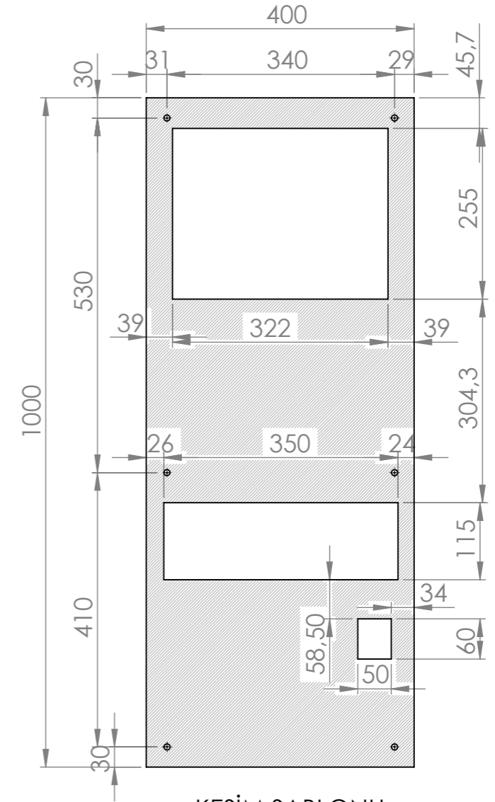
KESİM ŞABLONU
