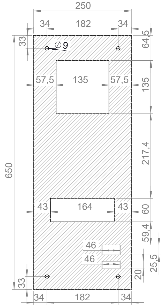
KESİM ŞABLONU CUTTING TEMPLATE
