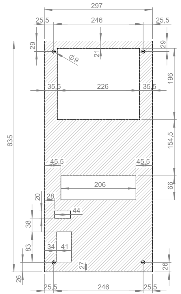
KESİM ŞABLONU CUTTING TEMPLATE
