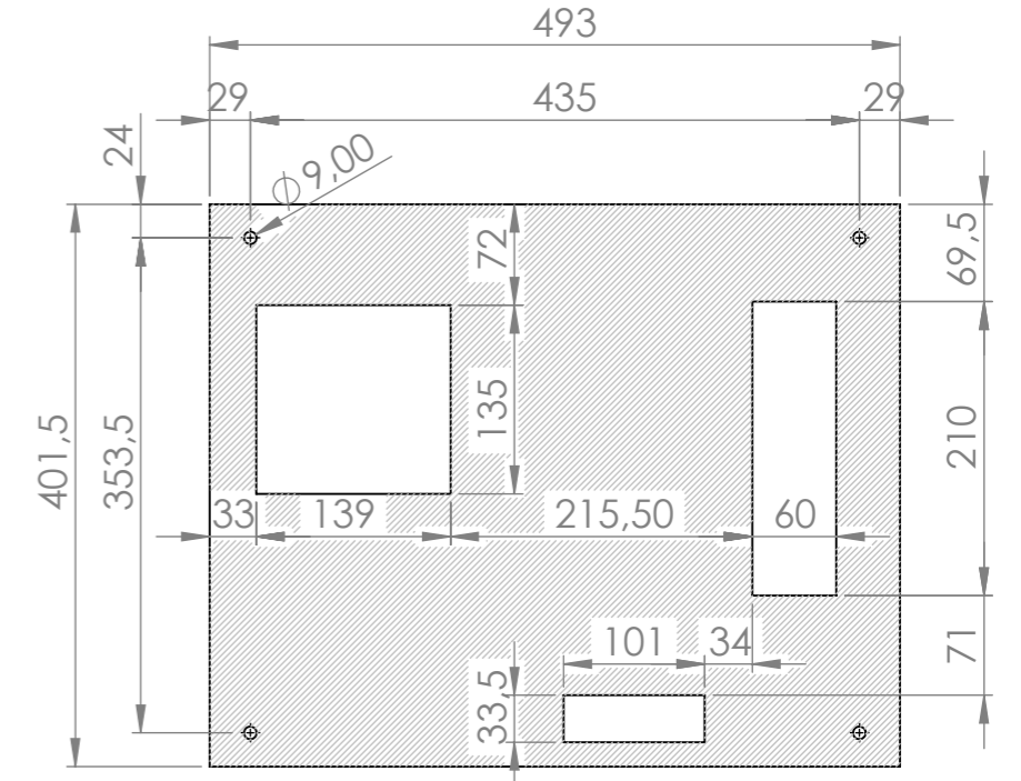
KESİM ŞABLONU CUTTING TEMPLATE
