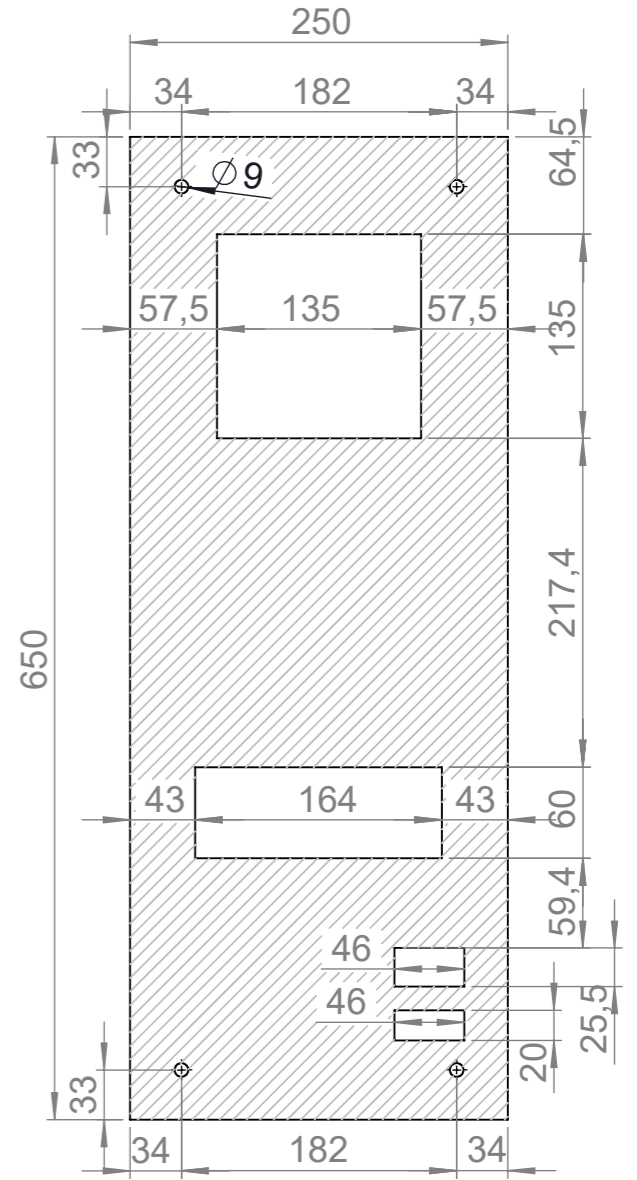
KESİM ŞABLONU CUTTING TEMPLATE
