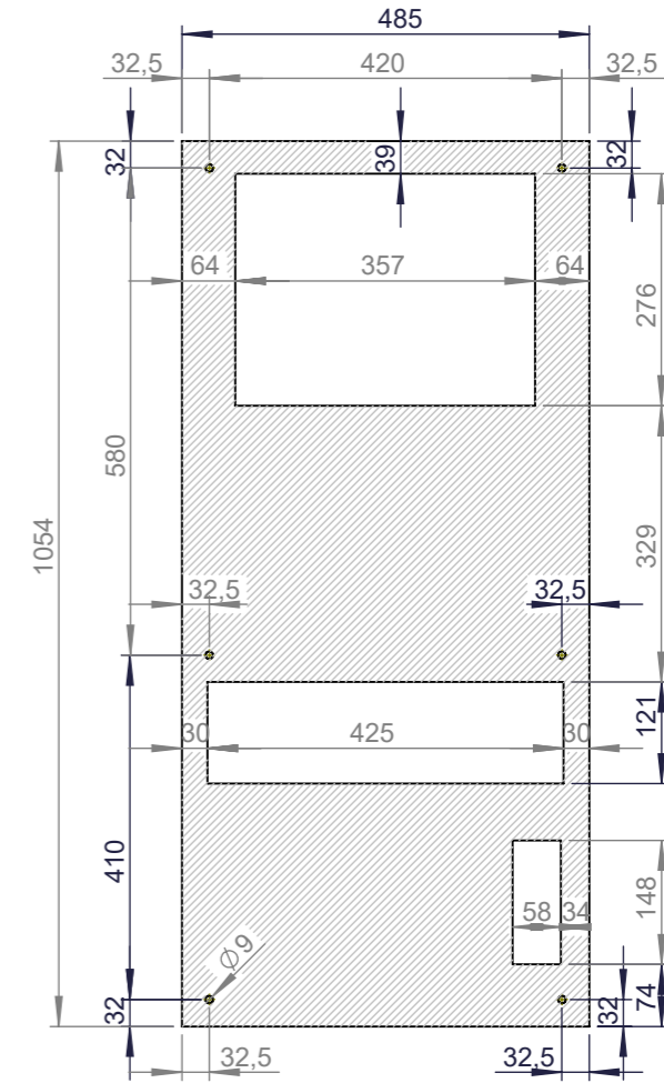
KESİM ŞABLONU CUTTING TEMPLATE
