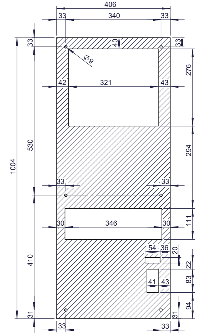
KESİM ŞABLONU CUTTING TEMPLATE
